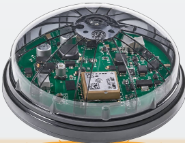
عقدة LiDAR من D-SLS على قاعدة D4i — Zhaga Book 18 · 20، يُثبت بالمشبك في أي وقت دون فتح جهاز الإنارة
